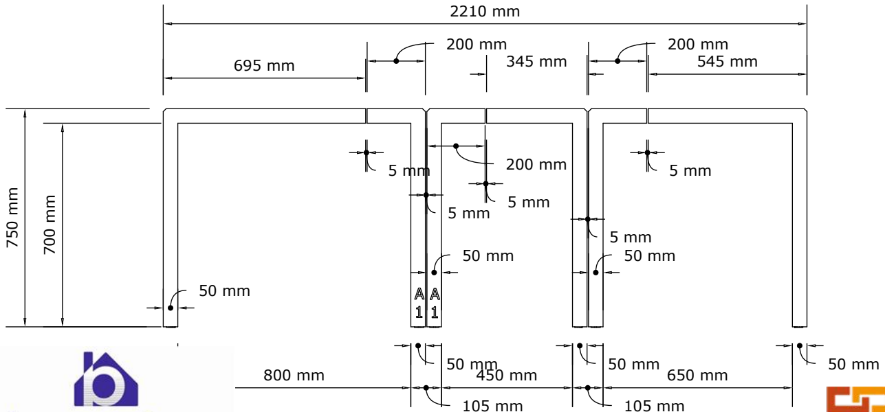
Grundriss Modul1 2.Reihe
