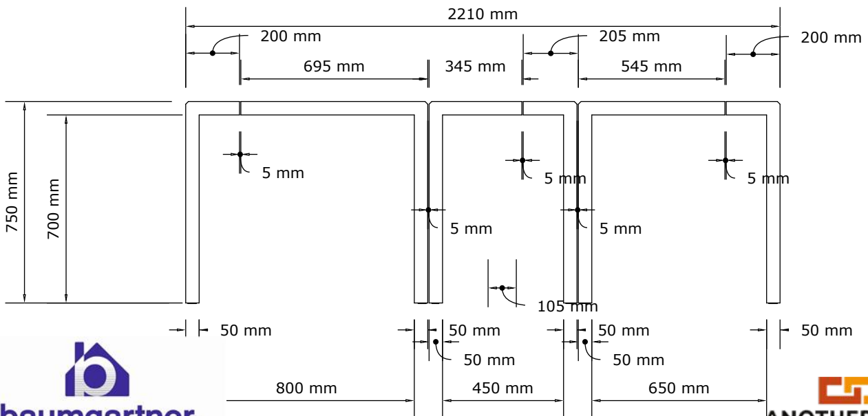
Grundriss Modul1 1.Reihe
